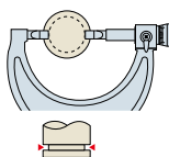
Mikrometer z ozkimi merilnimi konicami Za merjenje premerov znotraj ozkih utorov.
