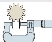
Zunanji mikrometer tipa disk Za merjenje tangent korena valjastih in vijačnih zobnikov.
